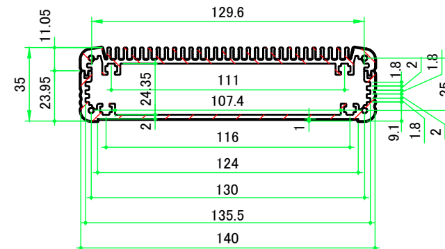
A-A (1:2.5)
